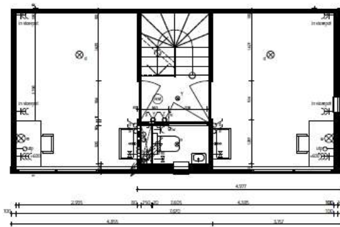
1e VERDIEPING 1:50
