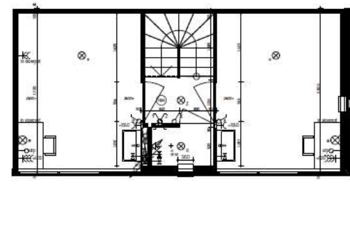
2e VERDIEPING 1:50
