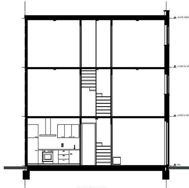
DOORSNEDE A
