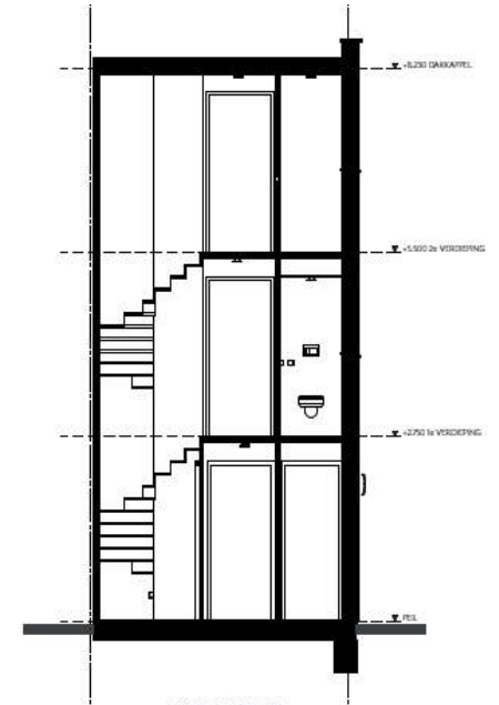
DOORSNEDE B1
