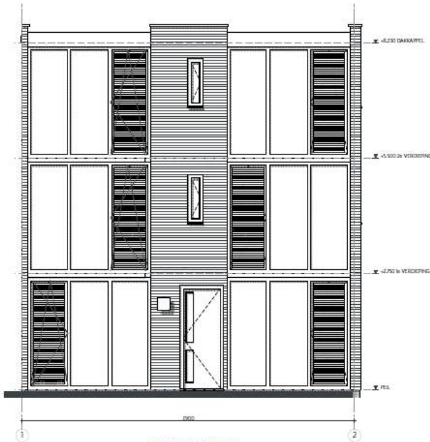
VOORAANZICHT 1:50
